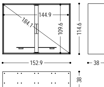
FREEDOM-TV 2 (FESTE RÜCKWAND)
