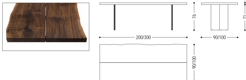
DETAIL: PLATTE AUS ZWEI PLANKEN
