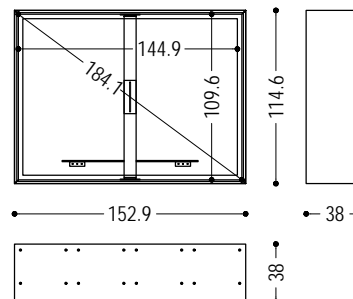
FREEDOM-TV 2-REV (DREHBARE RÜCKWAND)
