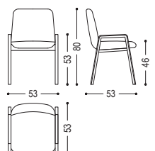
NOBLÉ' CHAIR CM: L. 53 · P. 53 · H. 46/80
