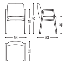
NOBLÉ' CHAIR.1 CM: L. 53 · P. 53 · H. 46/80
