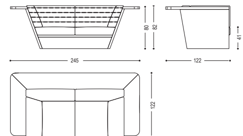
DYNAMIK 245 CM: L. 245 · P. 122 · H. 41/82
