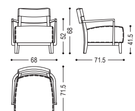
WILMA / B CM: L. 68 · P. 71,5 · H. 41,5/68
