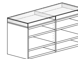
Modulo singolo con ripiani e teca superiore, EN Single unit with shelves and glass display case
