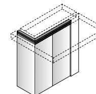
Pannello fisso ad incasso, EN Recessed fixed panel
